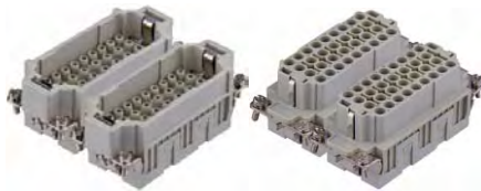
HEE-064-MC HEE-064-FC
